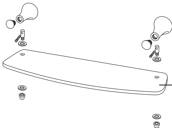
VIDRO PRATELEIRA INNOVARE CPD.03666
